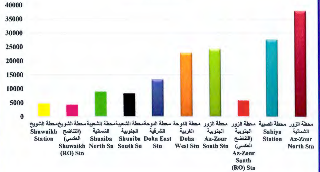
إجمالي الناتج Gross Production
