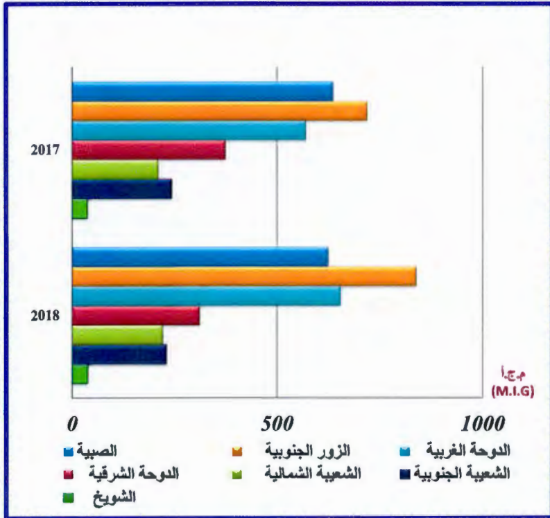
اجمالي مياه تعويض الغلايات Boilers Feed Water Make-Up
