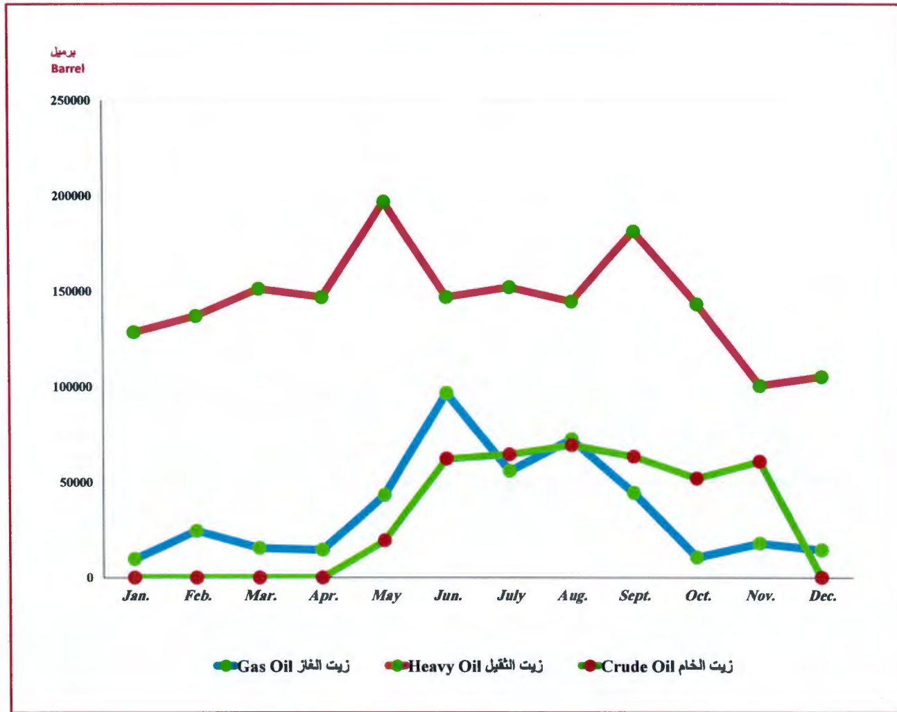
أعلى إستهلاك يومي من الوقود السائل ( برميل ) في محطات القوى الكهربائية وتقطير المياه خلال عام ٢٠١٨ Maximum Daily Consumption of Liquid Fuel by P/D Plants ( Barrels ) During 2018
